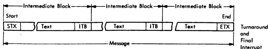
Figure 21. ITB Message
